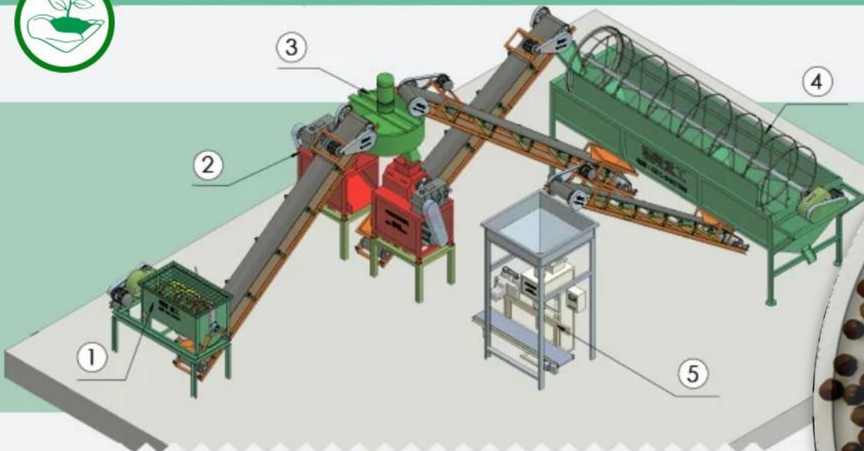
1. Смеситель 2. Гранулятор 3. Дисковый измельчитель 4. Просеиватель гранул 5. Фасовочный узел
